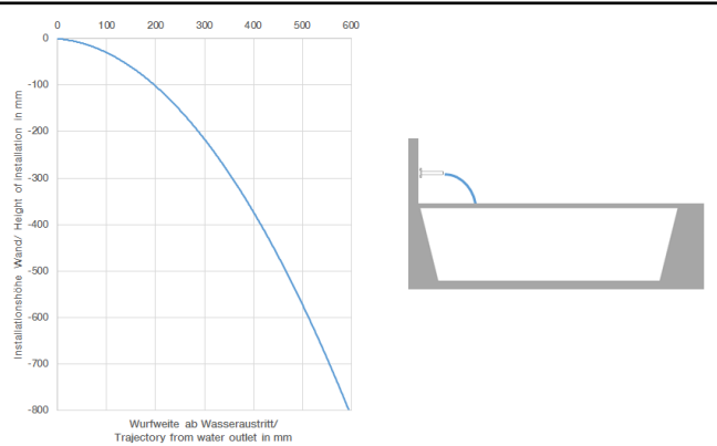
Wurfweitendiagramm
